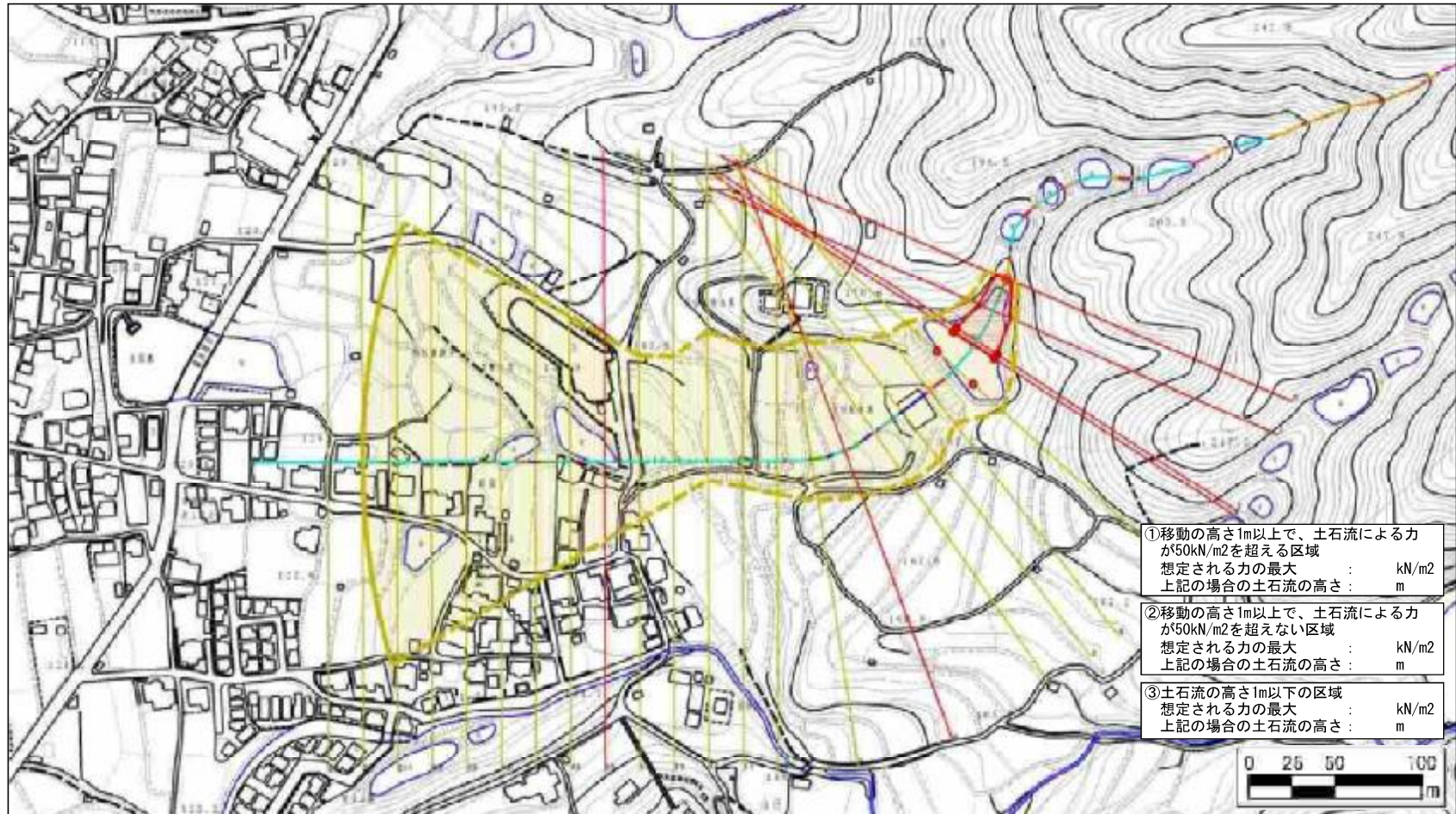
様式-3 (土) 土砂災害警戒区域等 区 域 図
