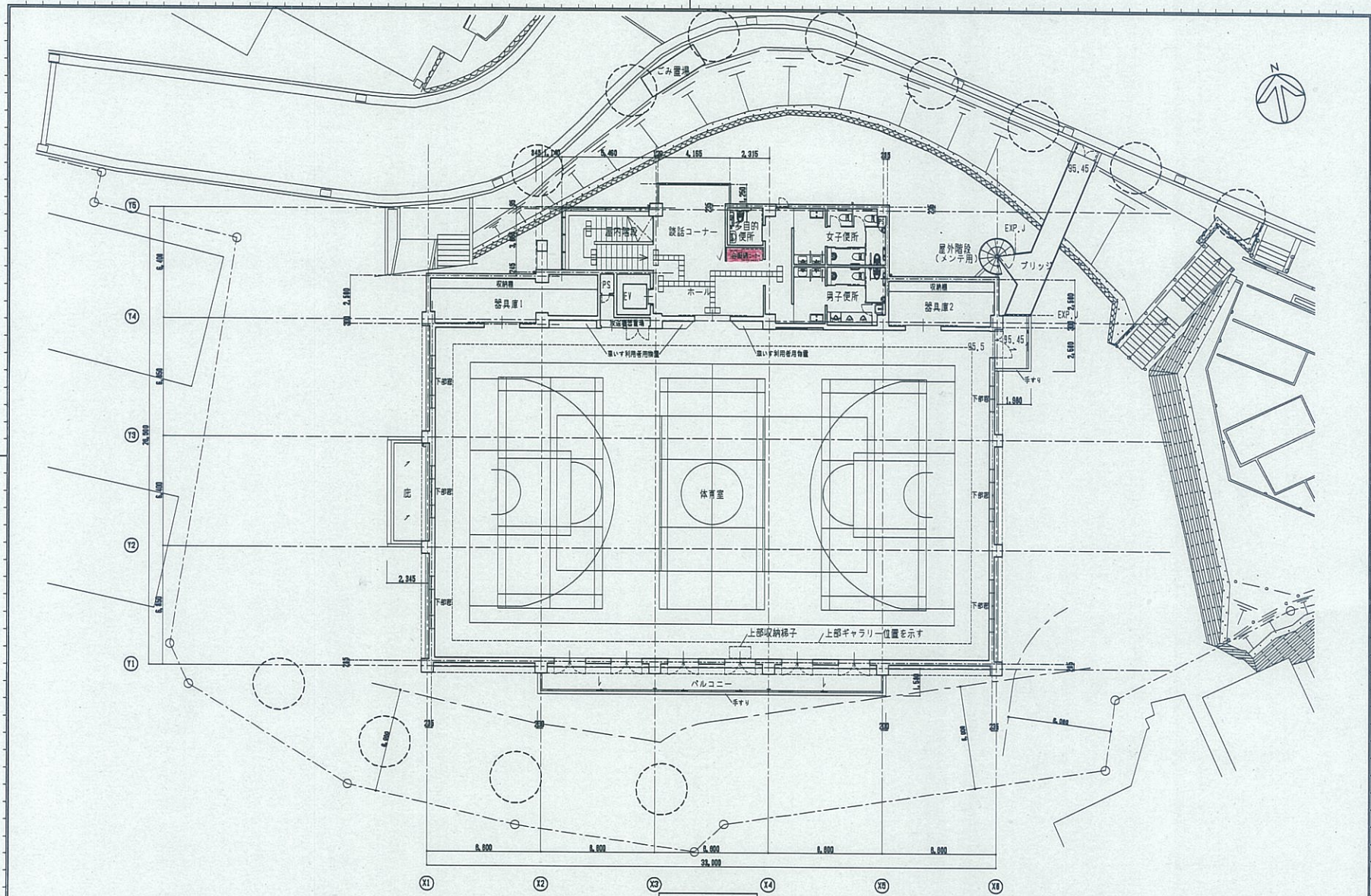
2階平面図 ②=1/100
