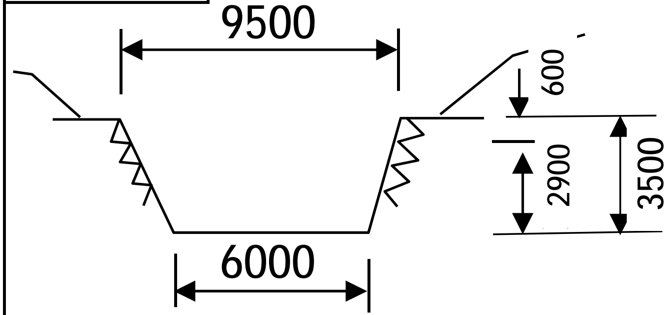
標準断面図
