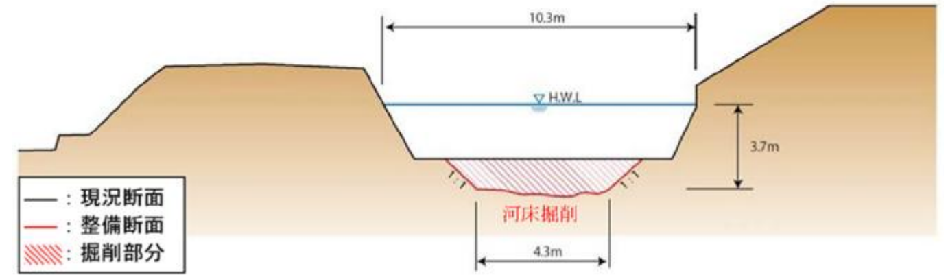
整備断面例 (5.6km 付近)
