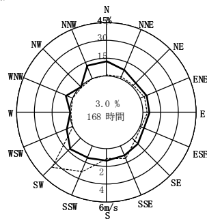
風配図（泉大津基地）〔令和元年8月分〕
