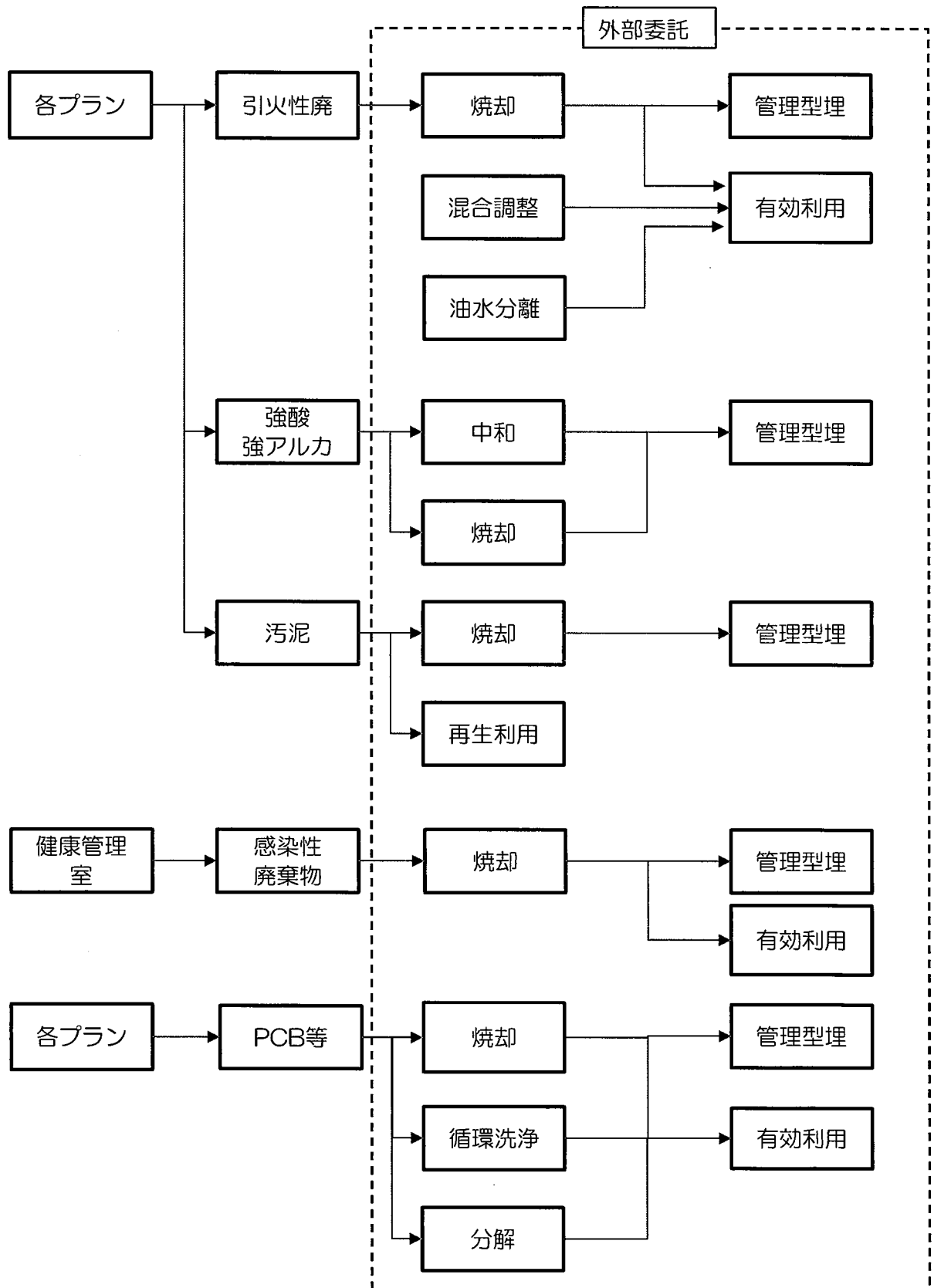
特別管理産業廃棄物処理工程図
