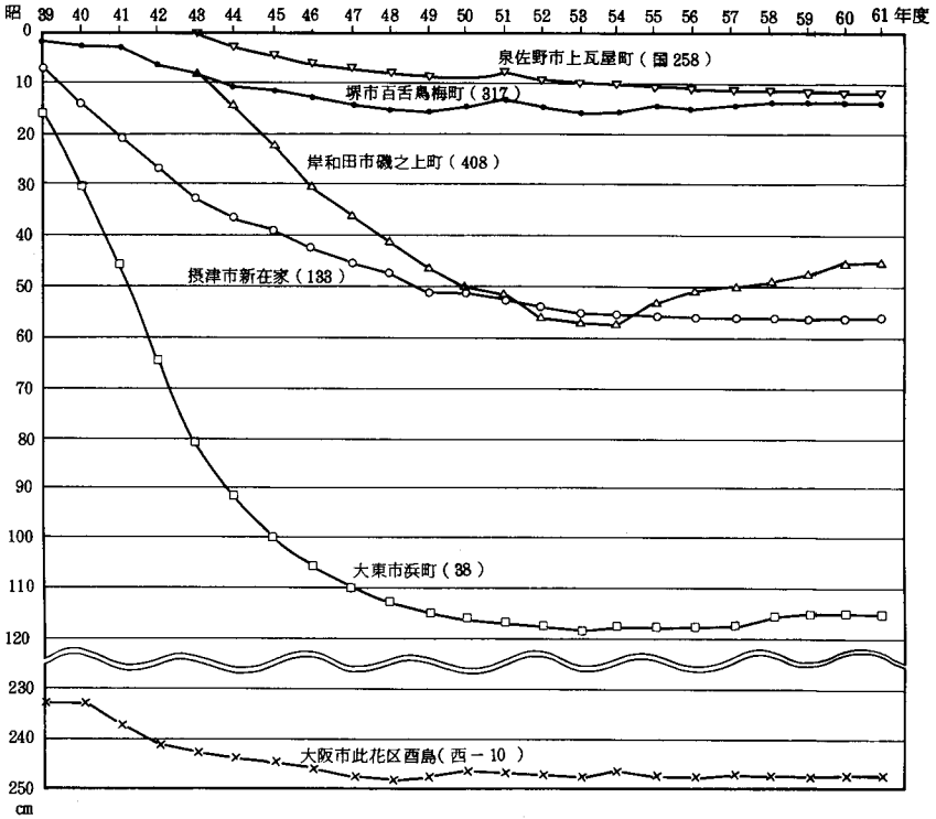
図 2-7-1 地盤沈下の推移
