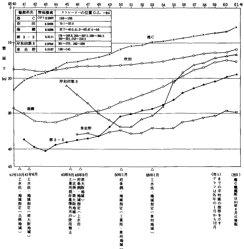
図2-7-2 地下水位の推移
