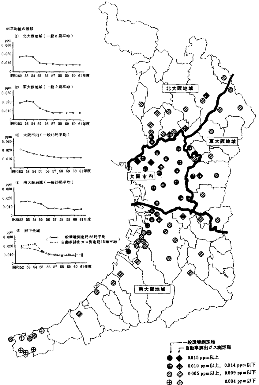
図2-2-1 二酸化硫黄濃度(年平均値)の概要(昭和61年度)と推移
