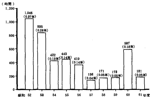
図2-2-15 昼間の光化学オキシダント濃度が0.12ppm以上の総時間数の推移
