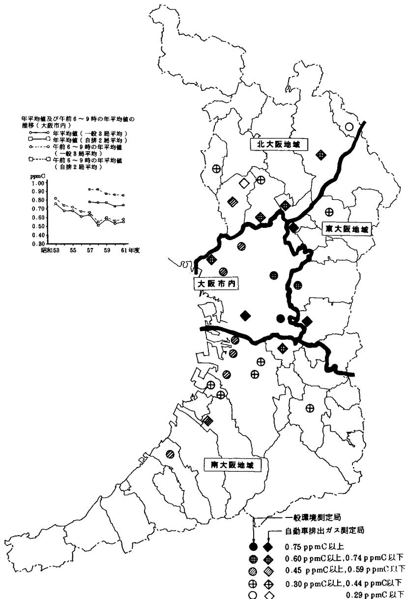
図 2-2-1 2 非メタン炭化水素濃度（年平均値）の概要（昭和 61 年度） と推移（年平均値及び午前 6～9 時の年平均値）
