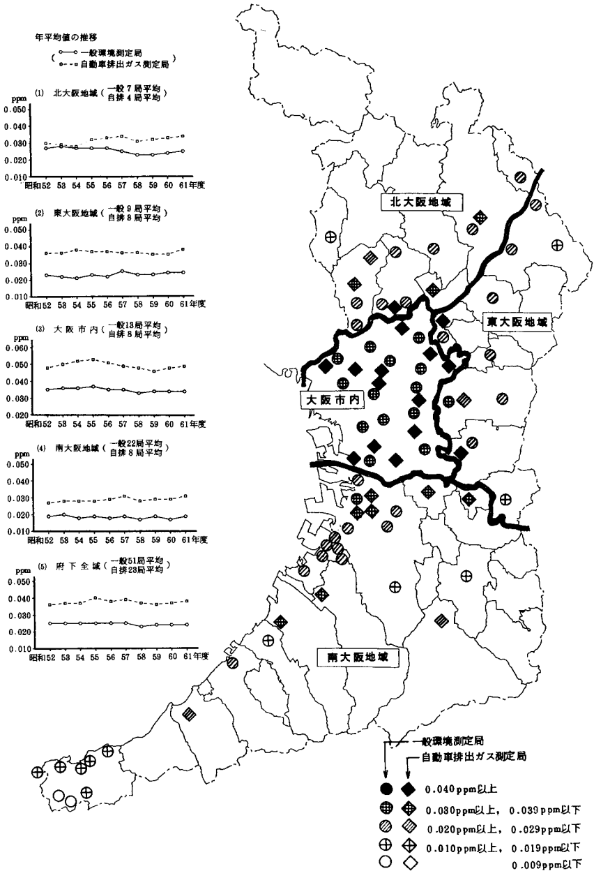
図2-2-3 二酸化窒素濃度(年平均値)の概要(昭和61年度)と推移
