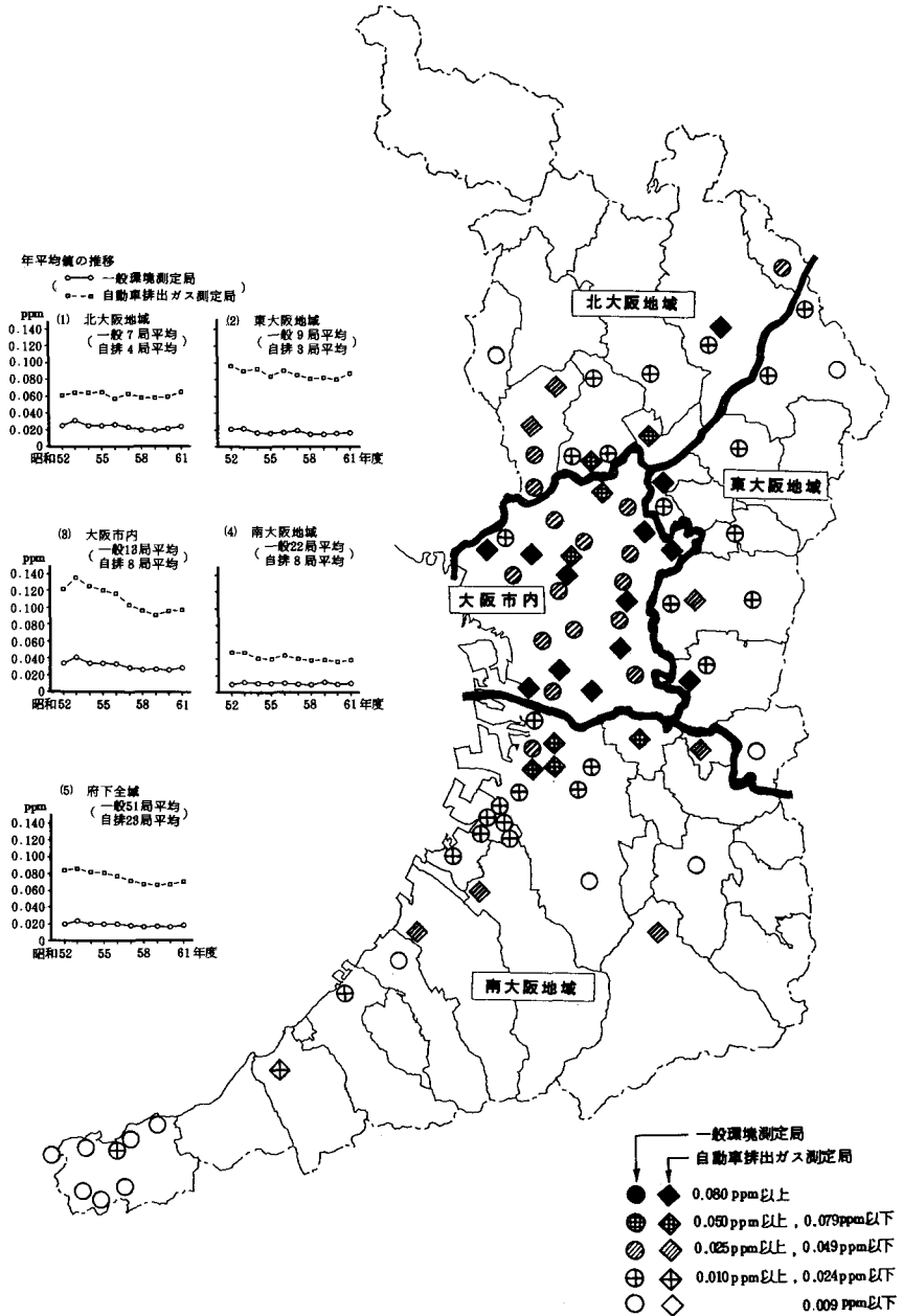
図 2-2-6 一酸化窒素濃度（年平均値）の概要（昭和 61 年度）と推移
