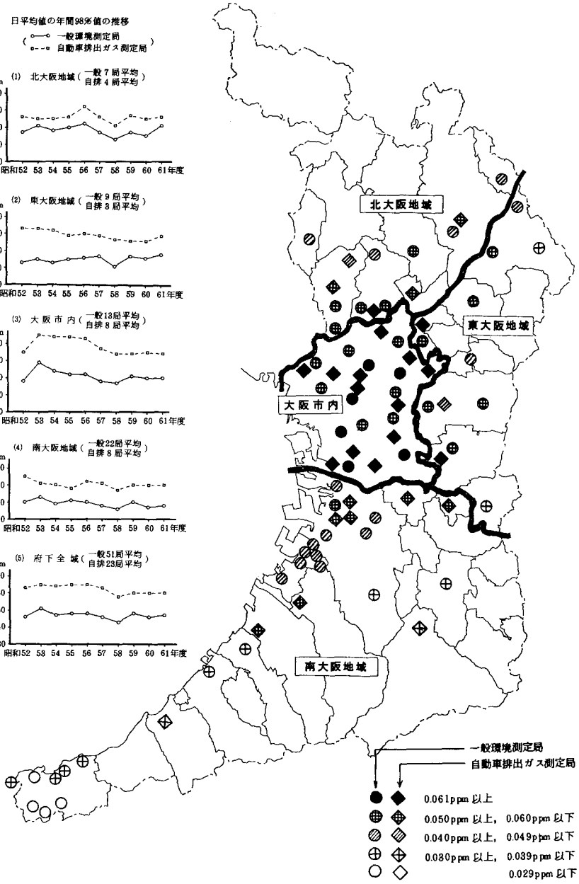
図 2-2-4 二酸化窒素濃度（日平均値の年間98％値）の概要（昭和61年度）と推移
