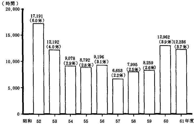
図2-2-14 昼間の光化学オキシダント濃度が0.06ppmを超えた総時間数の推移
