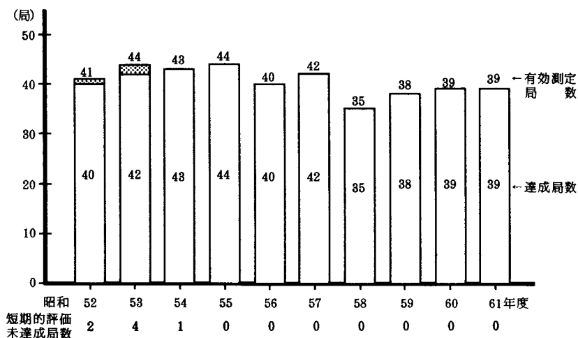
図 2 - 2 - 11 一酸化炭素濃度の環境基準達成状況（長期的評価）の推移
