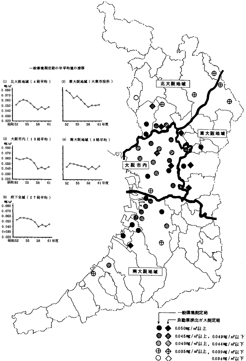
図 2-2-7 浮遊粒子状物質濃度（年平均値）の概要（昭和 61 年度）と推移
