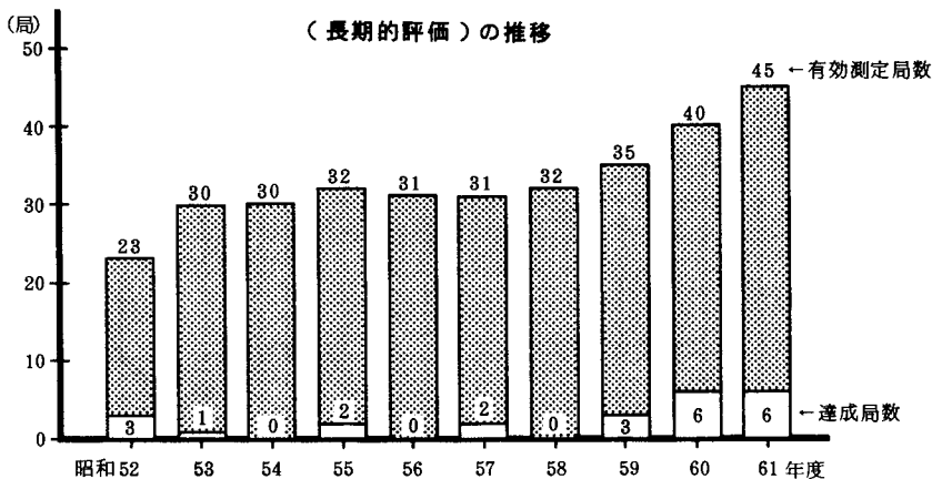
図 2-2-8 浮遊粒子状物質の環境基準達成状況
