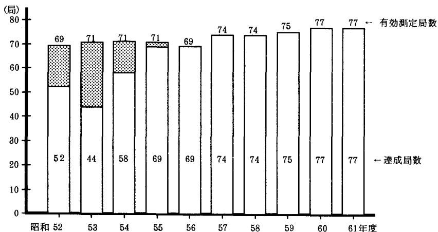
図 2-2-2 二酸化硫黄の環境基準達成状況（長期的評価）の推移
