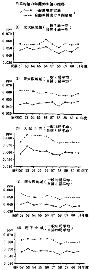
図 2-2-4 二酸化窒素濃度（日平均値の年間98％値）の概要（昭和61年度）と推移
