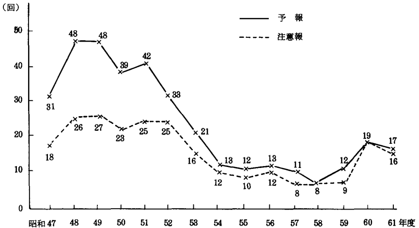
図 2-2-16 光化学スモッグ予報・注意報の発令回数の推移
