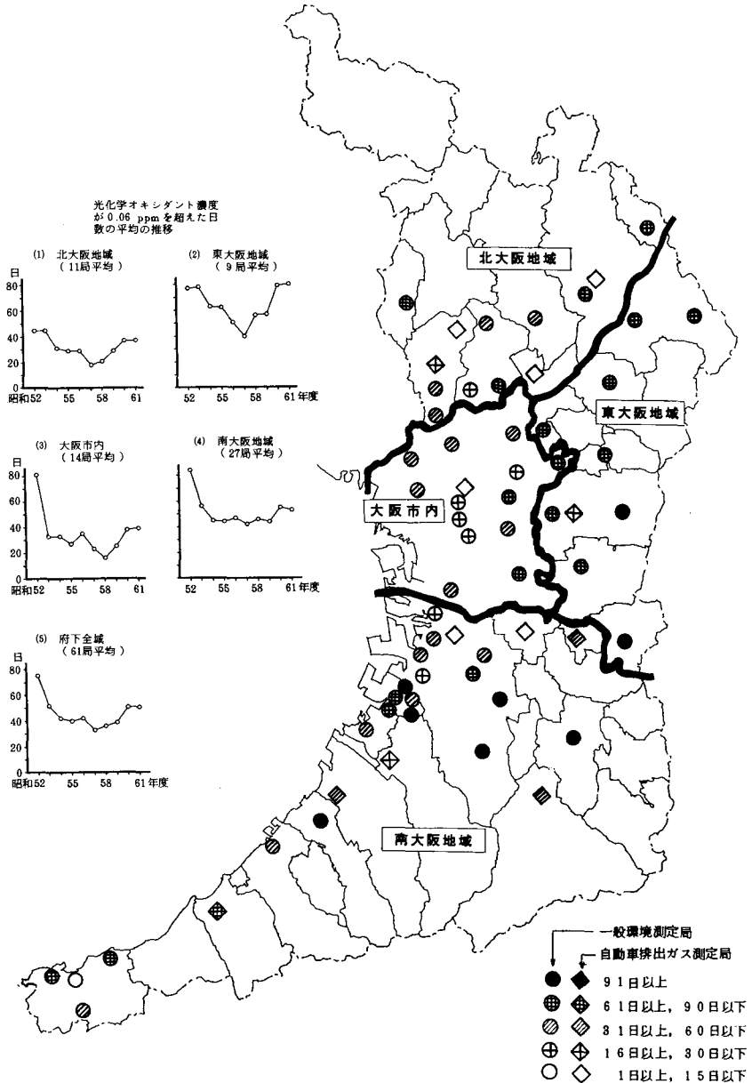
図 2-2-13 光化学オキシダント濃度が0.06ppmを超えた日数の概要(昭和61年度)と推移
