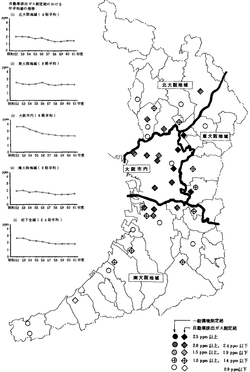
図 2-2-10 一酸化炭素（年平均値）の概要（昭和 61 年度）と推移
