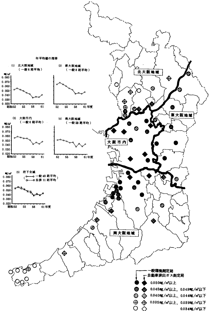
図2-2-9 浮遊粉じん濃度(年平均値)の概要(昭和61年度)と推移
