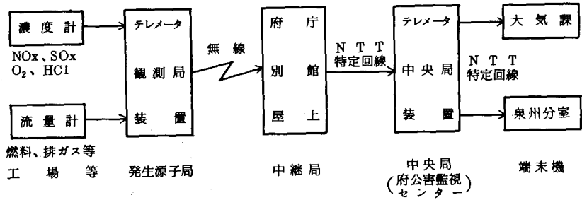
図2-5-23 大気汚染発生源常時監視システムの概要
