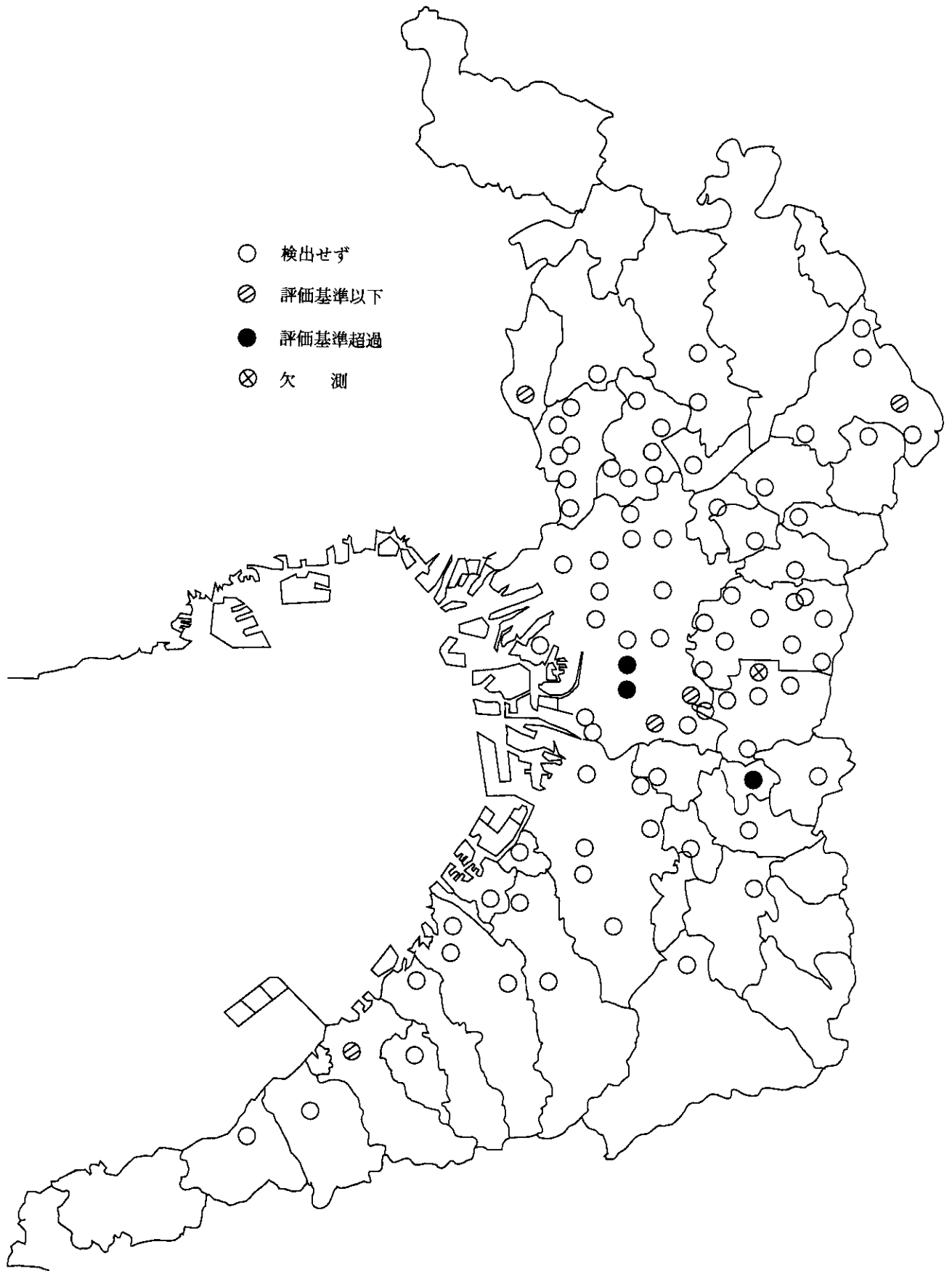
9-4 地下水質概況調査測定地点図 (平成5年度)
