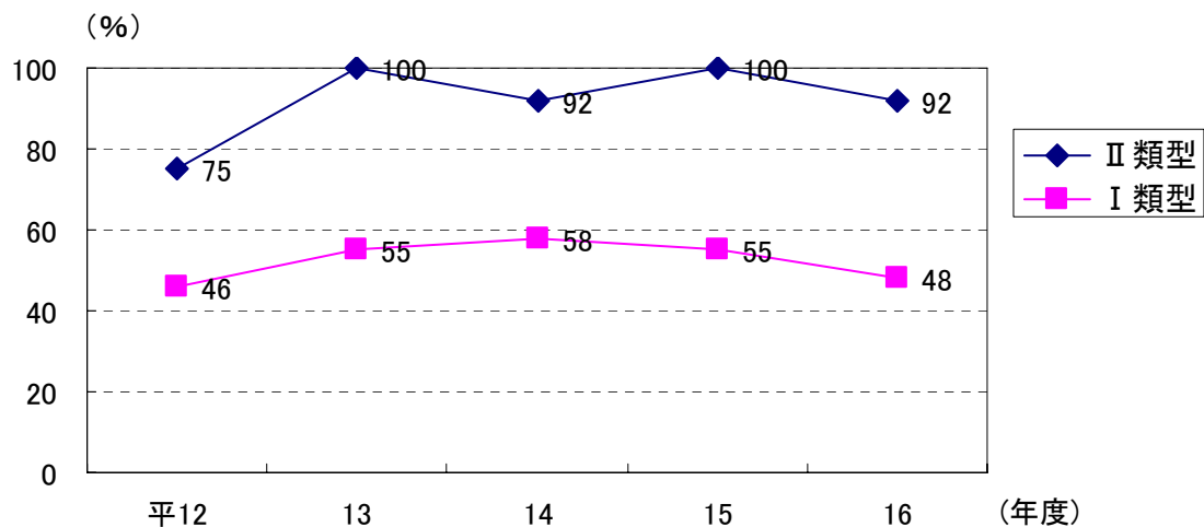
7-4 新幹線鉄道騒音の環境保全目標達成状況の推移
