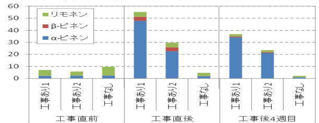
( \mu\text{g}/\text{m}^3 ) 香り成分 (テルペン類) —No.1
