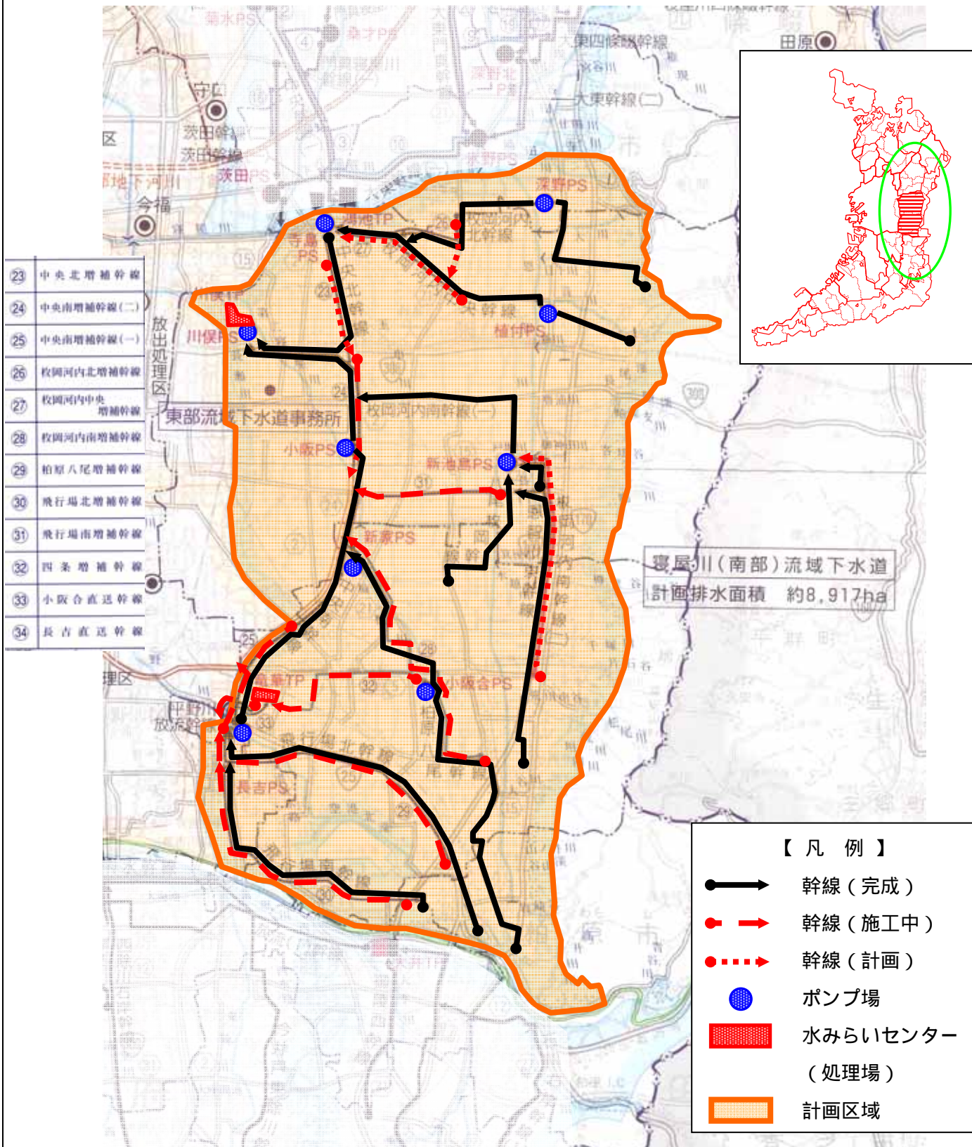
事業箇所図
