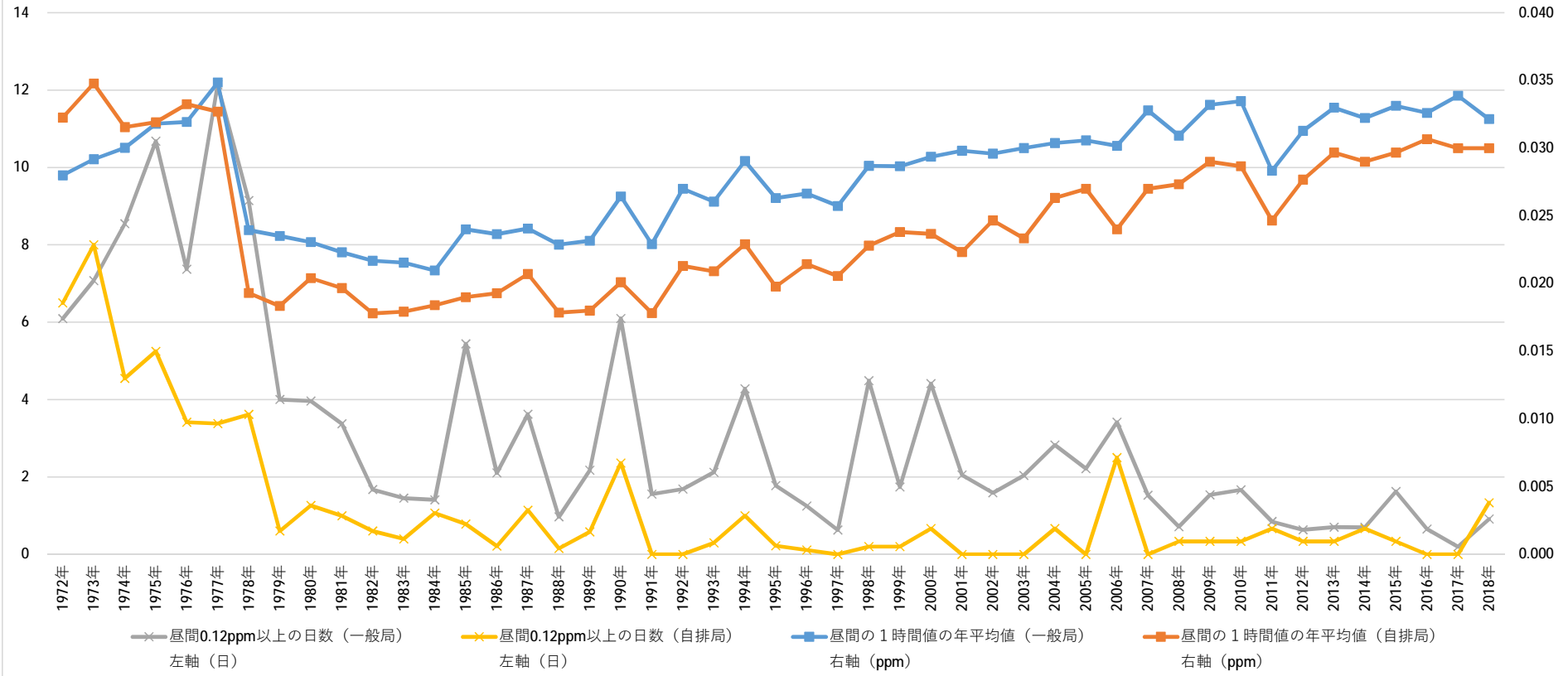
大阪府内におけるオキシダントの推移（1972～2018年）
