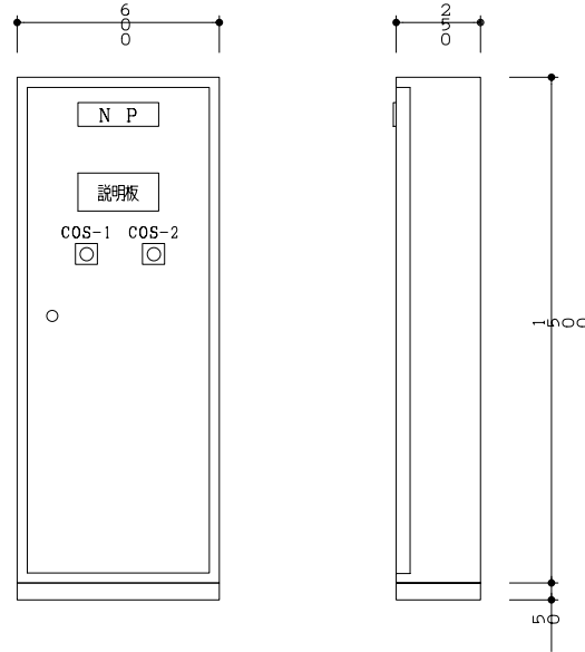
共用灯分電盤参考姿図
