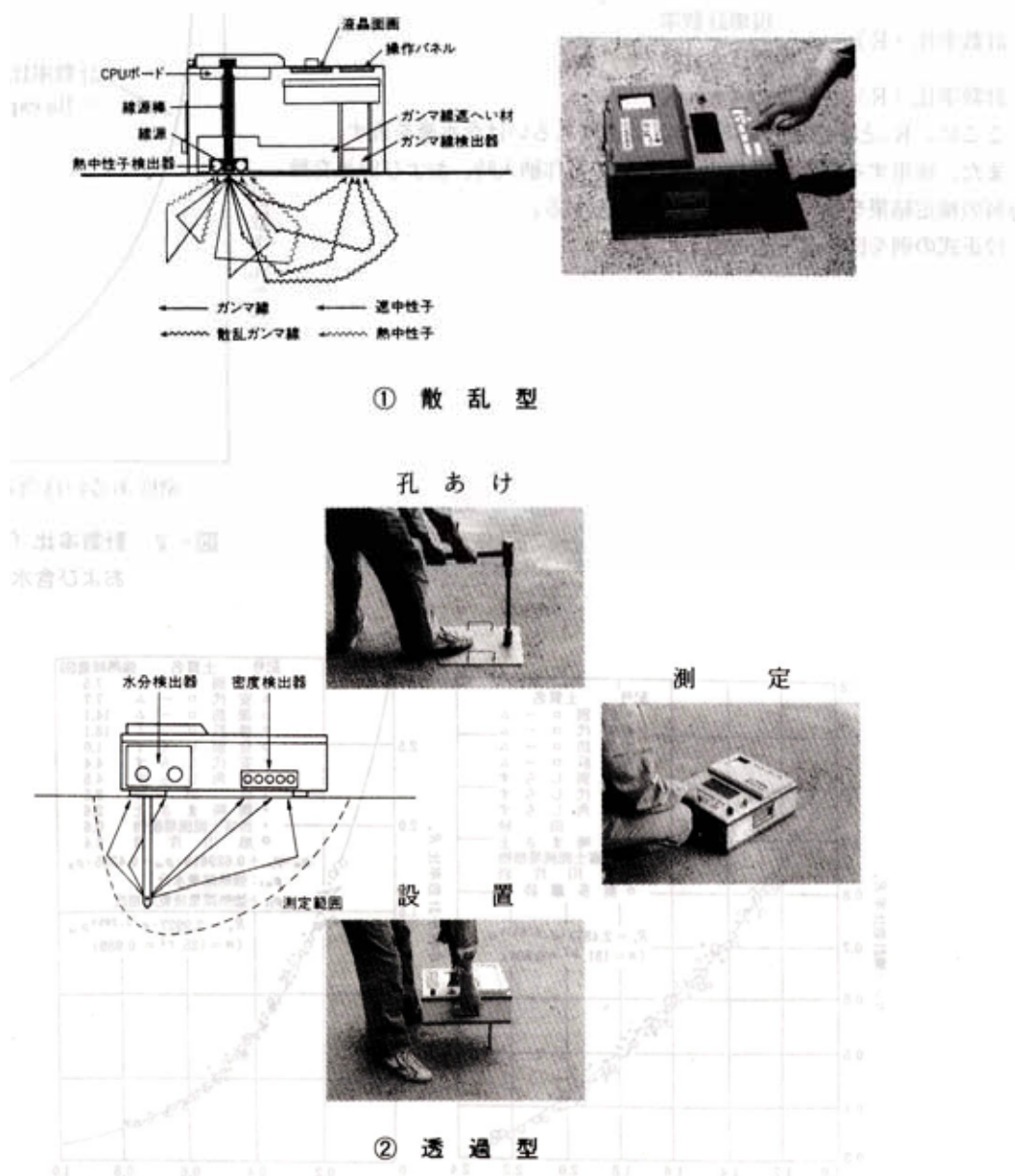
図 - 1 RI計器の概要
