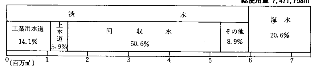
1日当り水源別工業用水使用量 (昭和47年)
