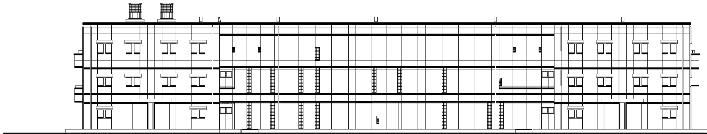
東 立 面 図 1/150
