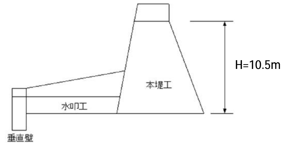
標準断面図
