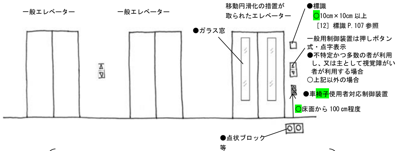
● 図 6.6 2台以上の場合の設計例
