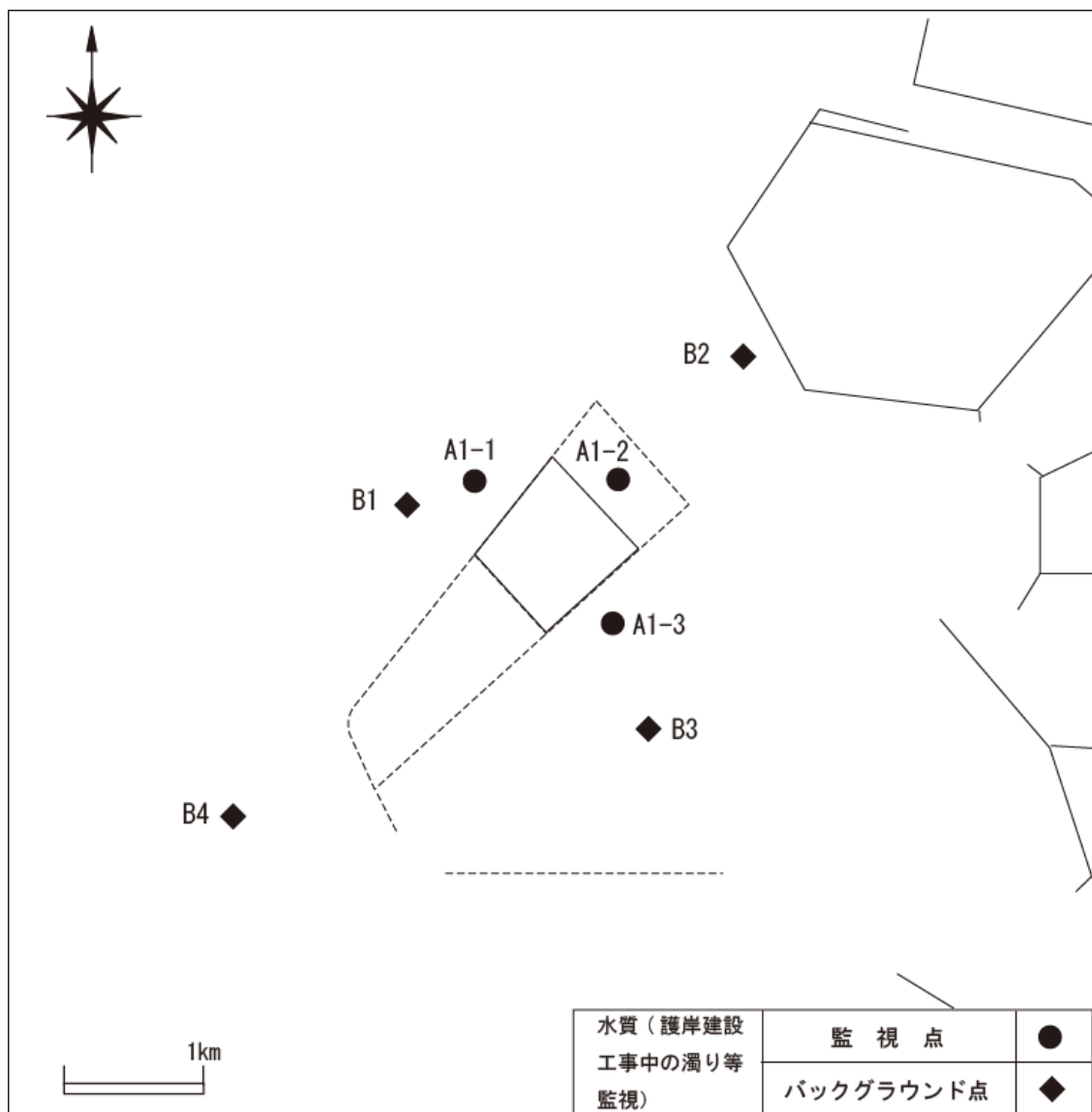
図一 1 (1) 調査地点(水質（護岸建設工事中の濁り等監視）)（平成 26 年度）
