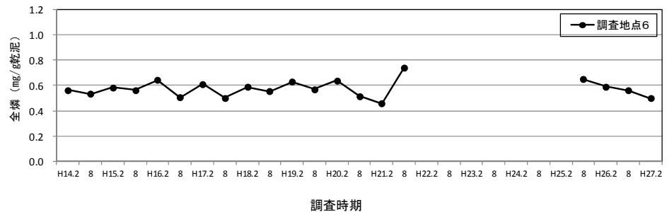
図－１５ 底質（化学的酸素要求量、硫化物、全窒素及び全燐）の経年変化
