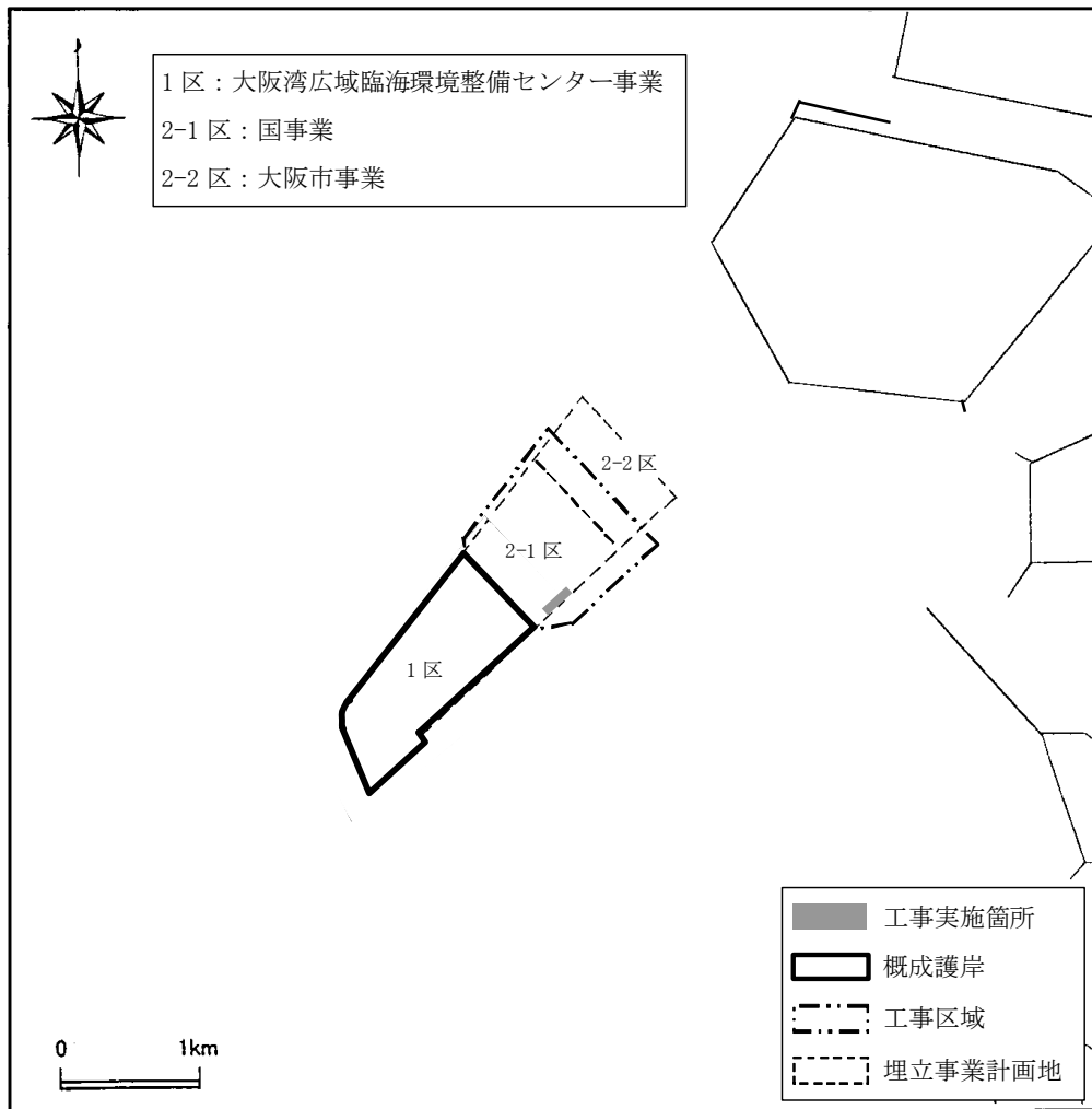
図-2(2) 工事の実施状況 (平成26年5月)
