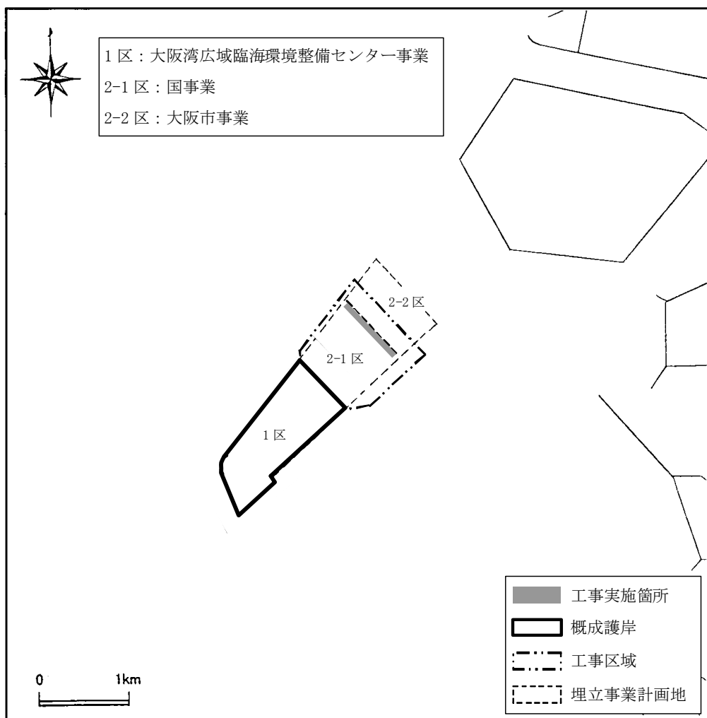
図-2(7) 工事の実施状況 (平成26年10月)
