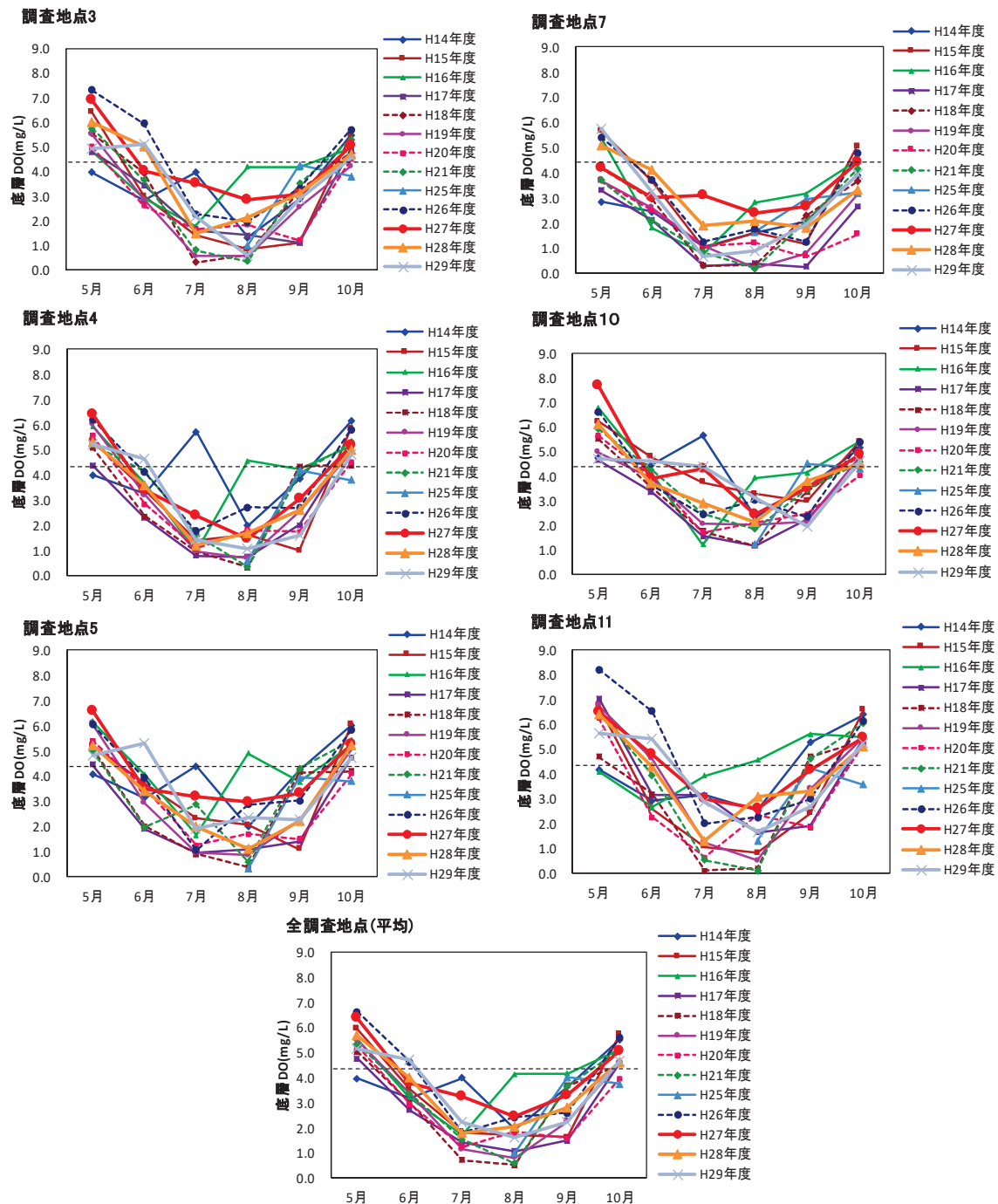
図-8 底層 D0 の過年度調査との比較
