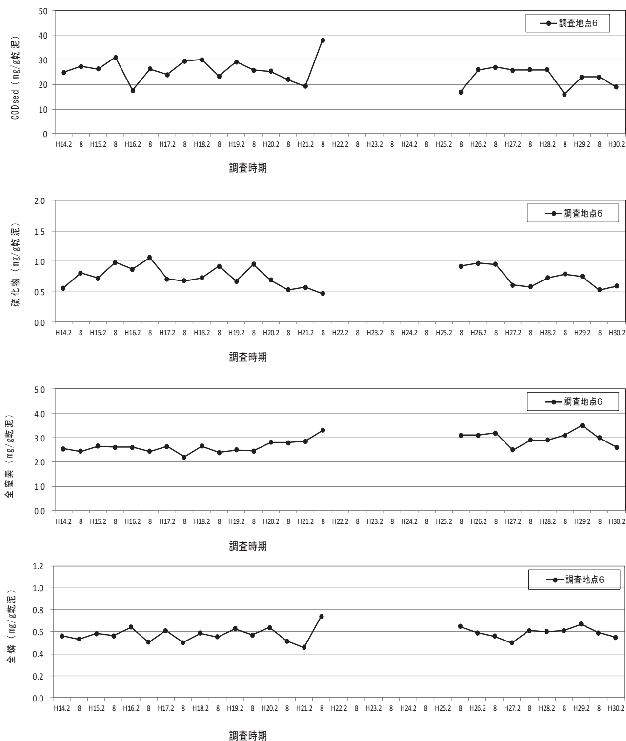
図-15 底質（化学的酸素要求量、硫化物、全窒素及び全燐）の経年変化
