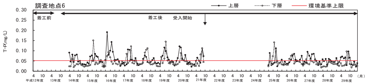
図-13 水質の経時変化
