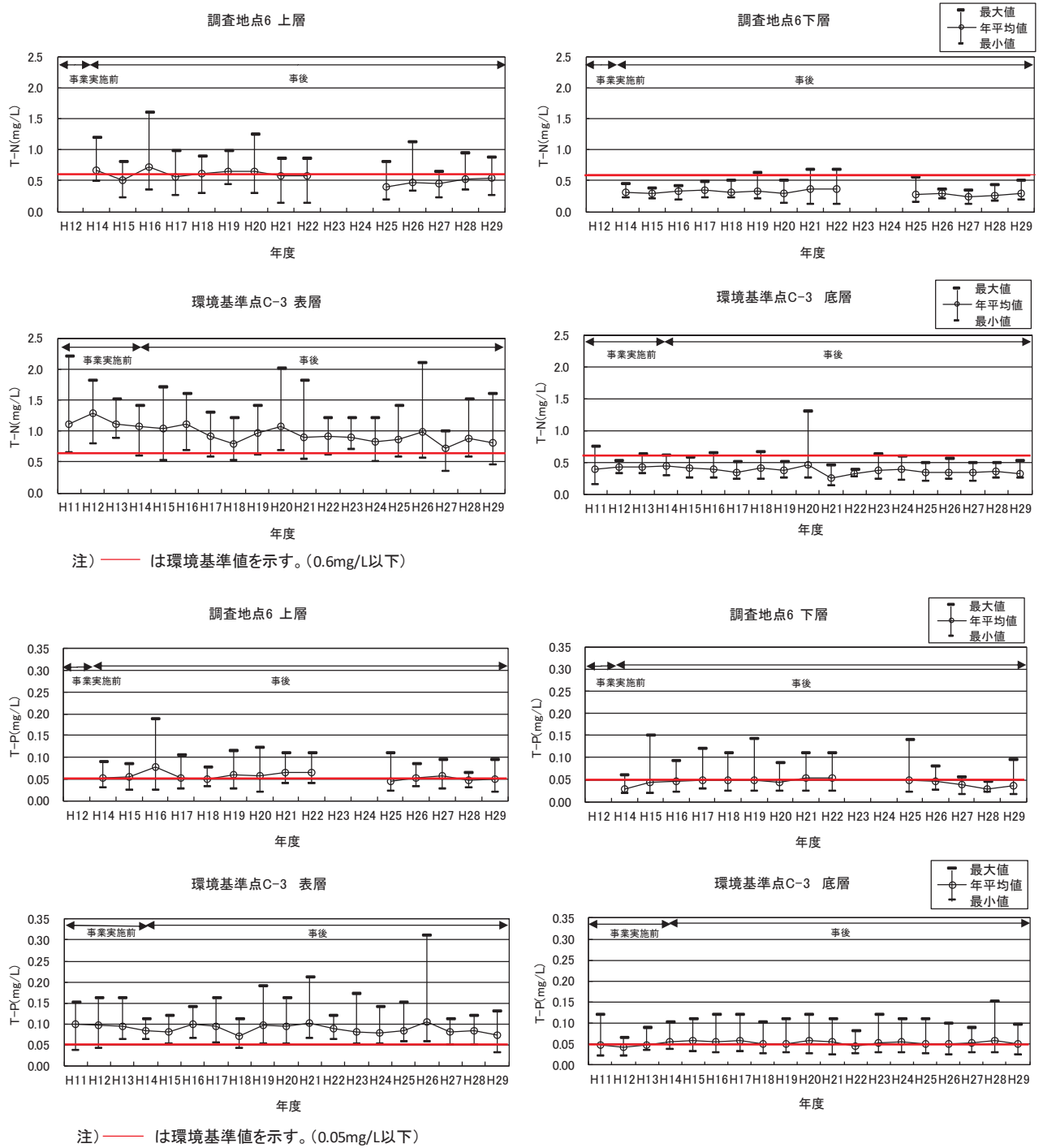
図-14(2) 環境基準及び事業実施前調査等との比較(水質：一般項目)
