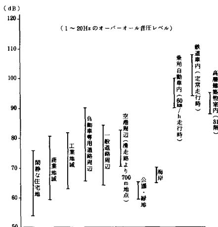
図2-4-8 生活環境における低周波空気振動音圧レベルの一例
