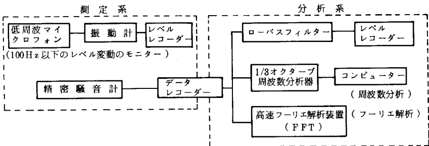
図 2-4-9 府における低周波空気振動の測定分析装置
