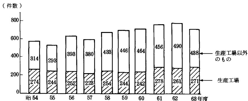
図1-1-6 悪臭の発生源別の推移
