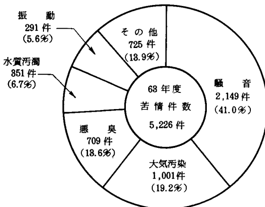
図1-1-5 公害の種類別苦情件数（昭和63年度）
